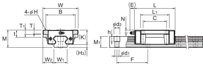
HSR85/LB型
