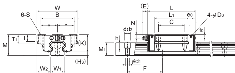
HSR20~35CA/HA/CAM/HAM型
