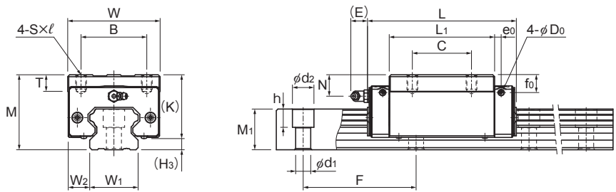
HSR45~85R/LR/XR/XLR型
