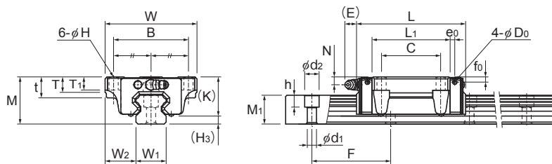
HSR20~35CB/HB/CBM/HBM型
