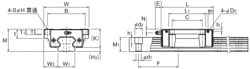
HSR45~65C/LC/XC/XLC型
