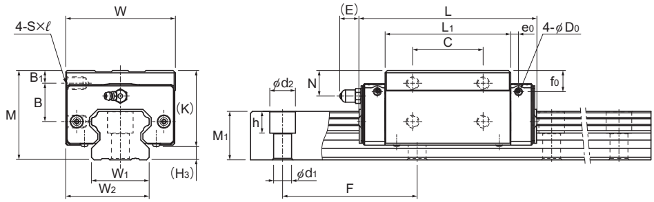
HSR45~65YR/XYR型
