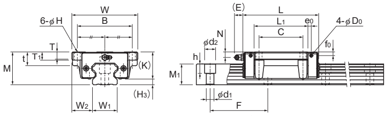
HSR45~85CB/HB/XCB/XHB型
