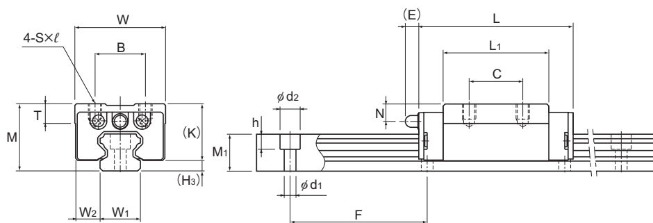
HSR12RM型
